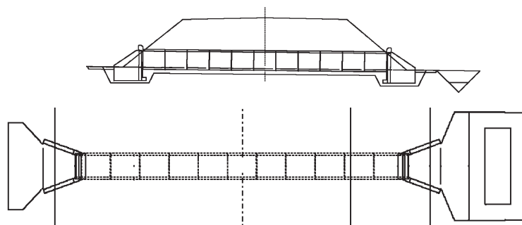
Рис. 46. Схема котлована под трубу и укрепление русел
