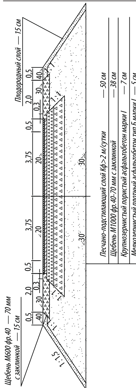
Рис. 27. Конструкция дорожной одежды
