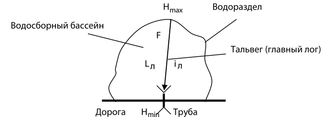
Рис. 30. План водосборного бассейна
