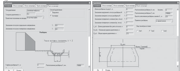
Рис. 45. Укрепление русла: а) основные данные; б) на входе; в) на выходе
