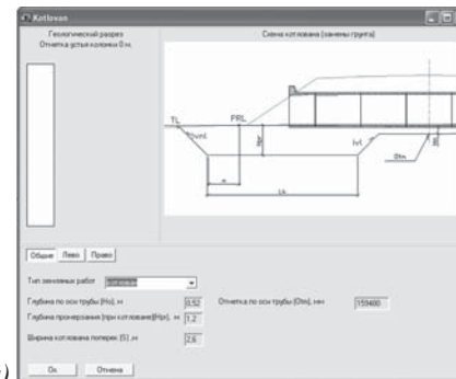
Рис. 44. Размеры котлована: а — общие по оси трубы;
