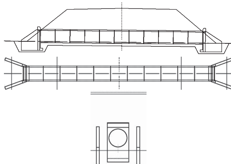
Рис. 43. Фасад, план и разрез с порталными и откосными стенками
